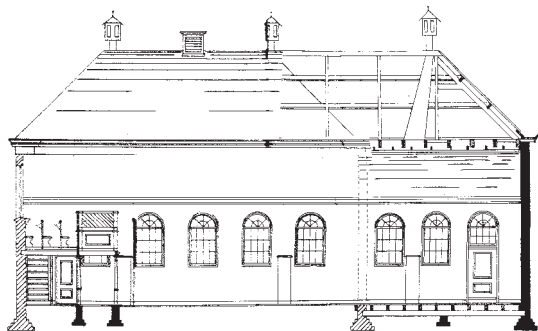
Verbouwingstekening uit 1900 van de Synagoge aan de Zeedijk. (coll. SAGV)
