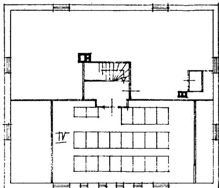
BEGANE GROND.
