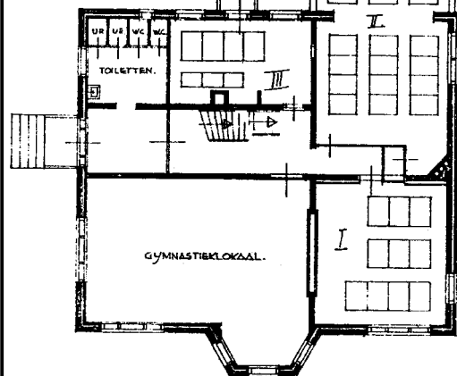
BEGANE GROND.
